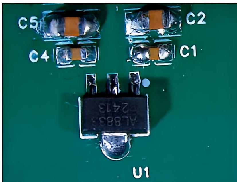
图 1 低压差线性稳压器-0006
